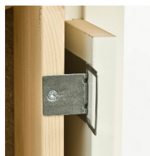
Monteringsbeslag for vindu med utforing.
